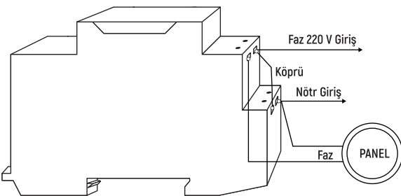
BAĞLANTI ŞEMASI
