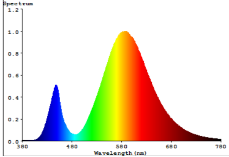
Grafik 1 : Tam yükte, 250 nm ile 800 nm aralığında Spektral Güç Dağıtımı Graph:1 : Spectral power distribution in the range 250 nm to 800 nm, at full-load
